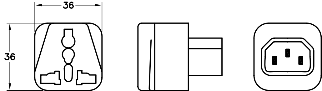
IEC 60320 C-14
